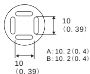
A1125B QFP 10x10 (0. 39x0. 39)
