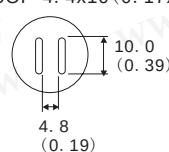
A1131 SOP 4. 4x10 (0. 17x0. 39)
