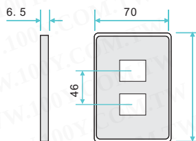
墙壁插座面板盖 卡式盖板2孔 尺寸: 120x70mm
