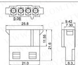
材料: nylon 66 UL94-2 F48 颜色: 白色
