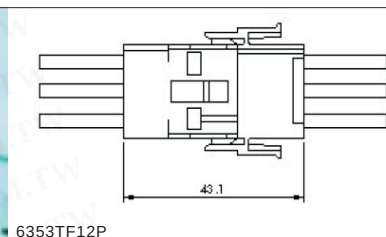
规格说明: 额定电流: 10A AC, DC (AWG 14) 最大电压值: 5000V AC/Minute 电阻阻力: 1000MΩ Min. 可适用PC 木板厚度: 1.6mm 额定电压: 600V AC, DC 接触电阻: 10mΩ Max. 操作温度: -55°C to +105°C
