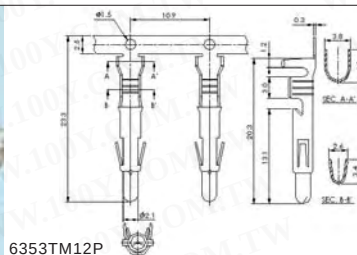
规格说明: 额定电流: 10A AC, DC (AWG 14) 承受电压: 5000V AC/Minute 绝缘电阻: 1000 mΩ Min 电压规定值: 600V AC, DC 接触电阻: 10mΩ Max 温度范围: -55°C to +150°C
