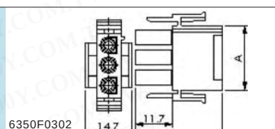
规格说明: 额定电流: 10A AC, DC (AWG 14) 最大电压值: 5000V AC/Minute 电阻阻力: 1000MΩ Min. 可适用PC 木板厚度: 1.6mm 额定电压: 600V AC, DC 接触电阻: 10mΩ Max. 操作温度: -55°C to +105°C
