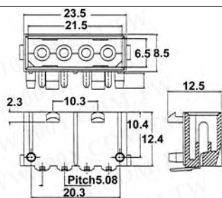
材料: Post: 黄铜, 锡/镀金 F53 Base: 尼龙 66, UL94V-2
