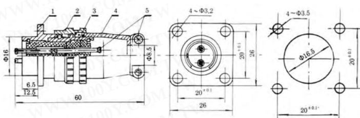
1. 凸缘壳体 2. 连接套 3. 壳体 4. 带翼套管 5. 螺钉
