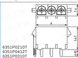
规格说明: 额定电流: 10A AC, DC (AWG 14) 承受电压: 5000V AC/Minute 绝缘电阻: 1000 mΩ Min 电压规定值: 600V AC, DC 接触电阻: 10mΩ Max 温度范围: -55°C to +150°C
