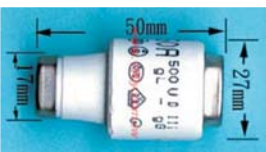
E27-10A-gL
