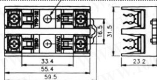
轨道保险丝座
