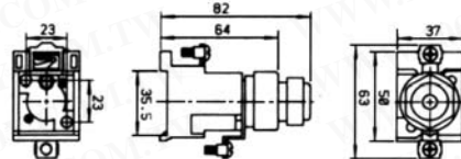
欧洲式 10*38 保险丝座(附灯)
