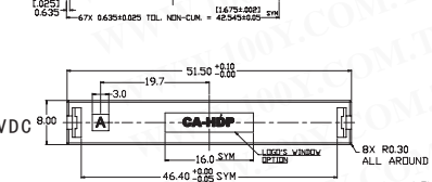
68LDP-A-P-1
