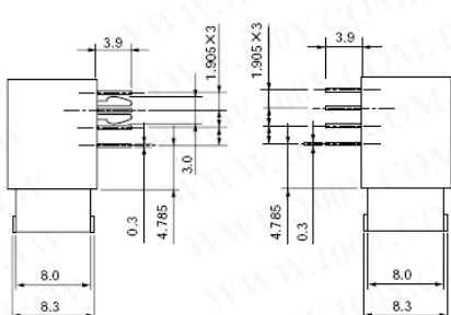
10150-52A2-JL
